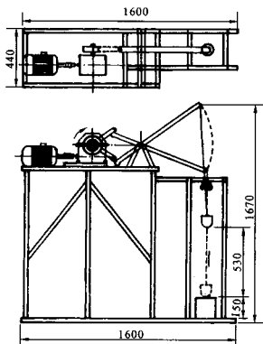
冲击试验仪
