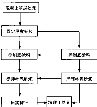
图 6.2 施工流程
