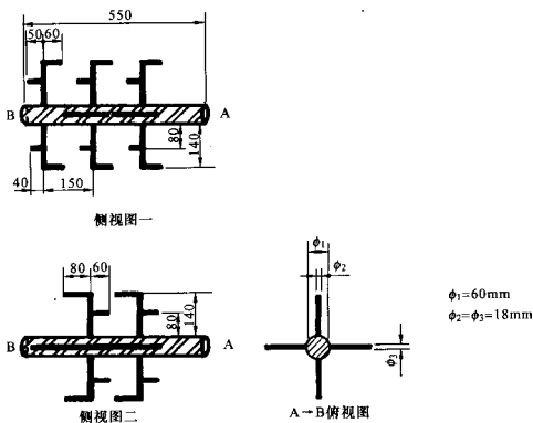
图 6.4.2-2 卧式拌和杆构造示意图
