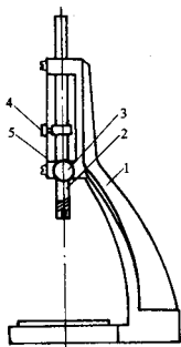
1—铁座；2—金属圆棒；3—松紧螺丝； 4—指针；5—标尺
